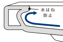
ボウル前面断面図
